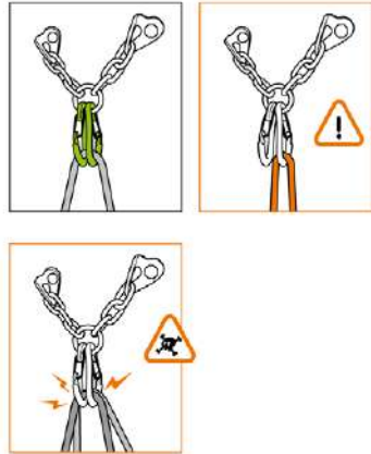
Installazione della corda sulla sosta per una moulinette
