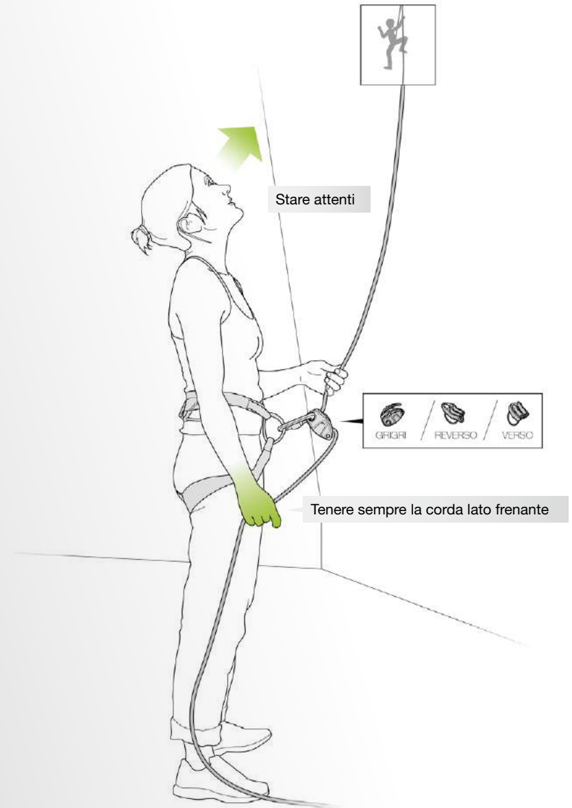
Principale posizione d'assicurazione
