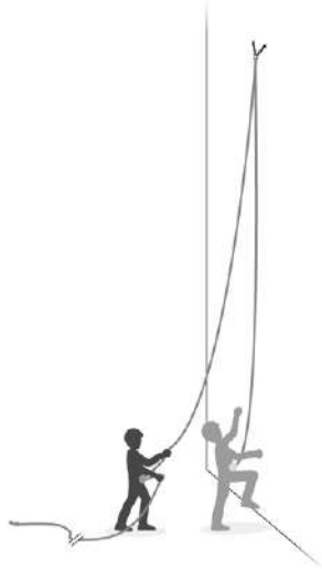
Moulinette con corda installata
